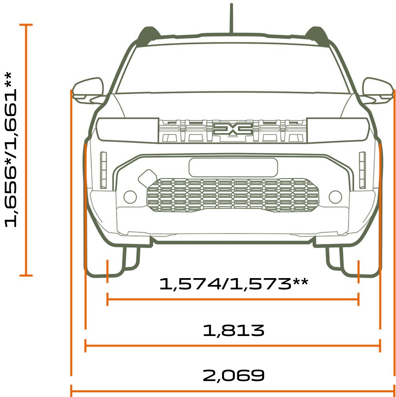
VISTA FRONTALE
