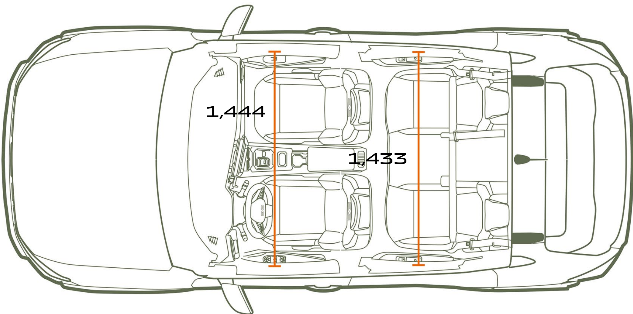
VISTA DALL'ALTO
