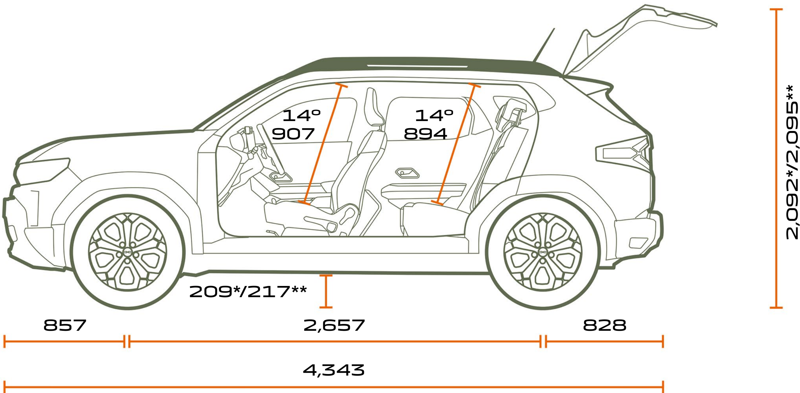
VISTA LATERALE
