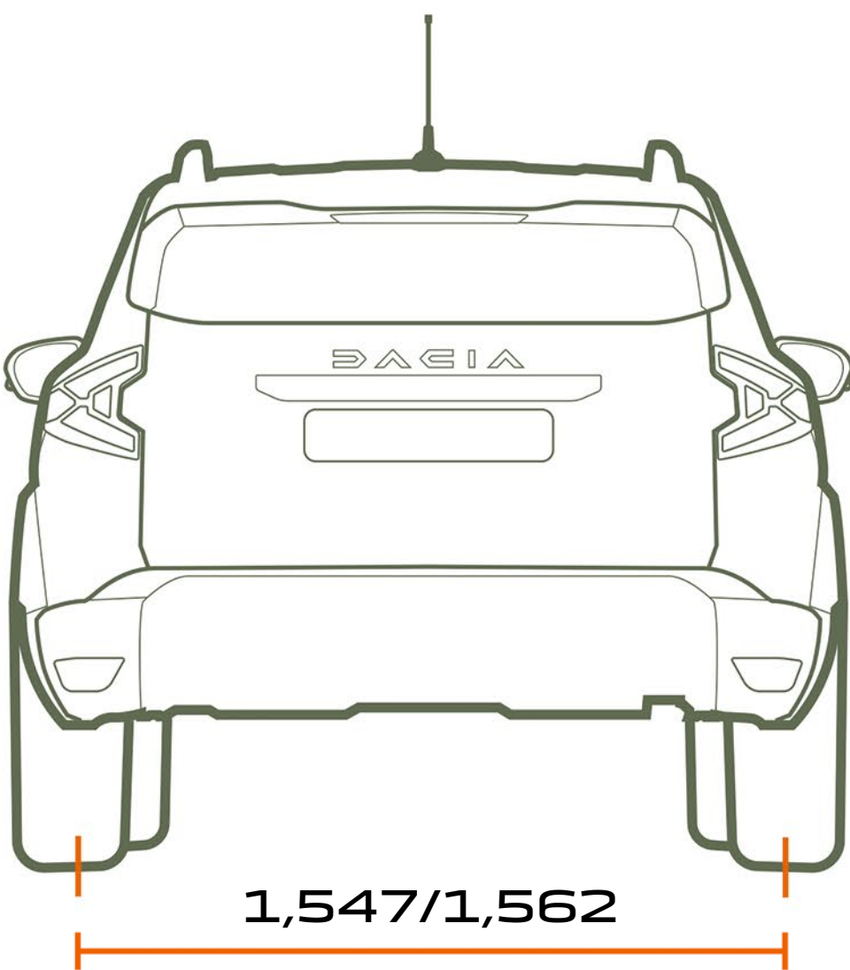
VISTA POSTERIORE
